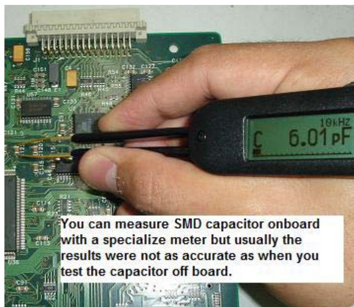
Smart Tweezers
